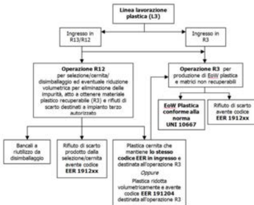
Schema a blocchi Linea di lavorazione plastica L3
