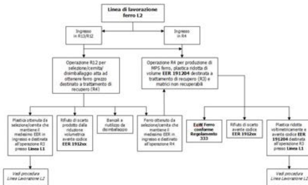
Schema a blocchi Linea di lavorazione ferro L2
