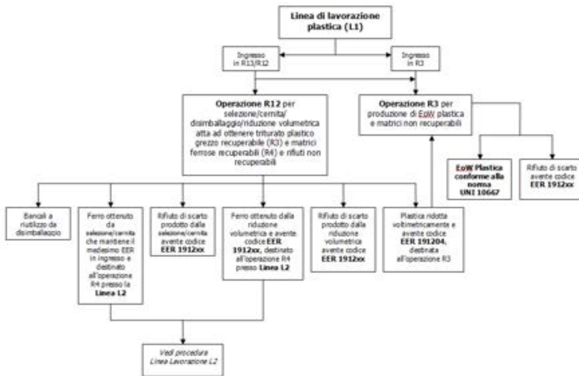
Schema a blocchi Linea di lavorazione plastica L1
