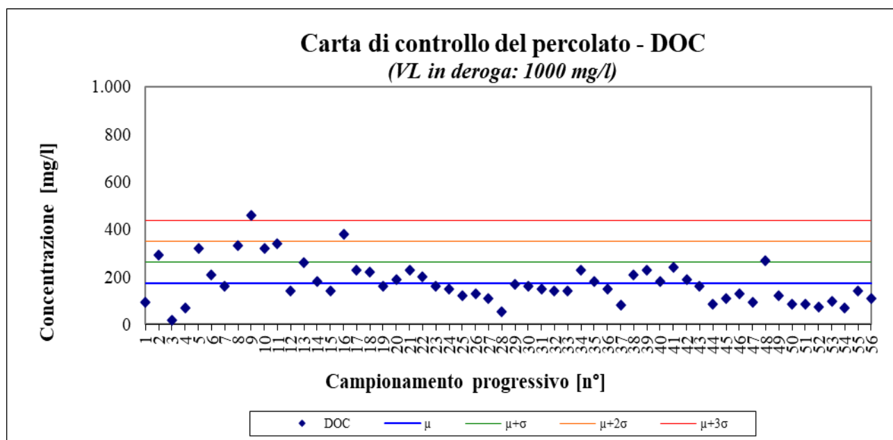
Figura 4 – DOC; periodo gennaio 2010 – ottobre 2023
