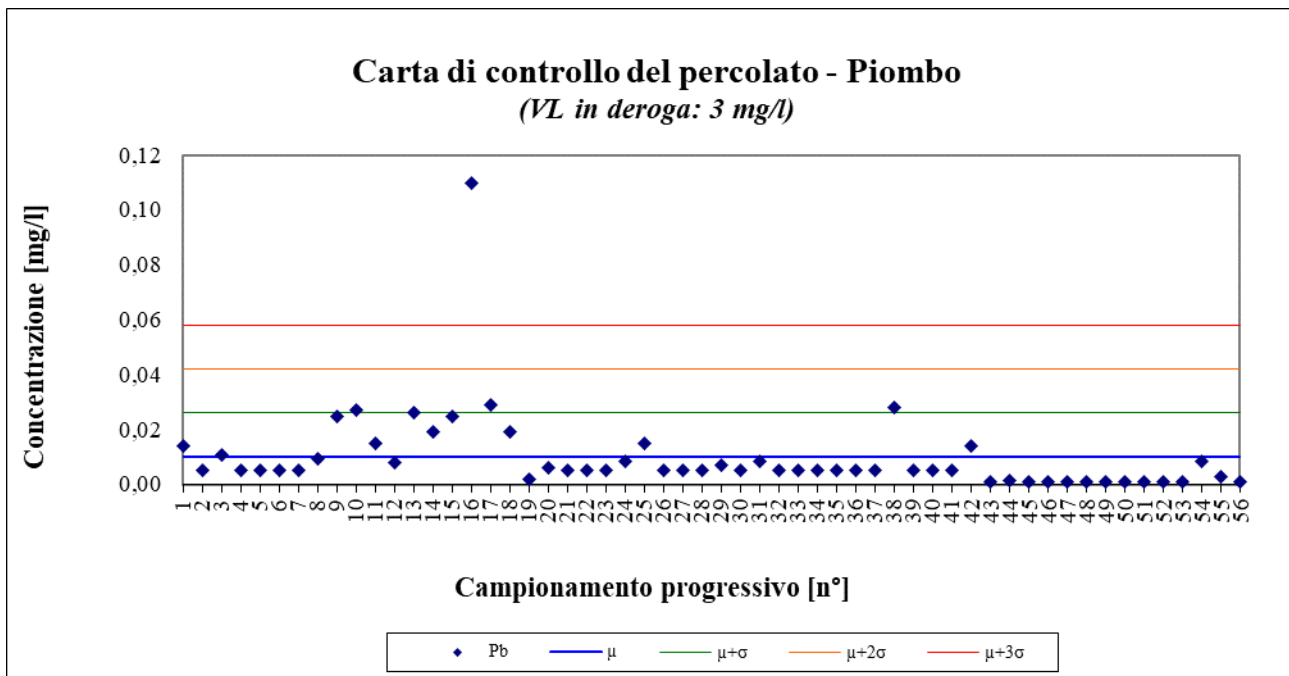
Figura 10 – Piombo; periodo gennaio 2010 – ottobre 2023
