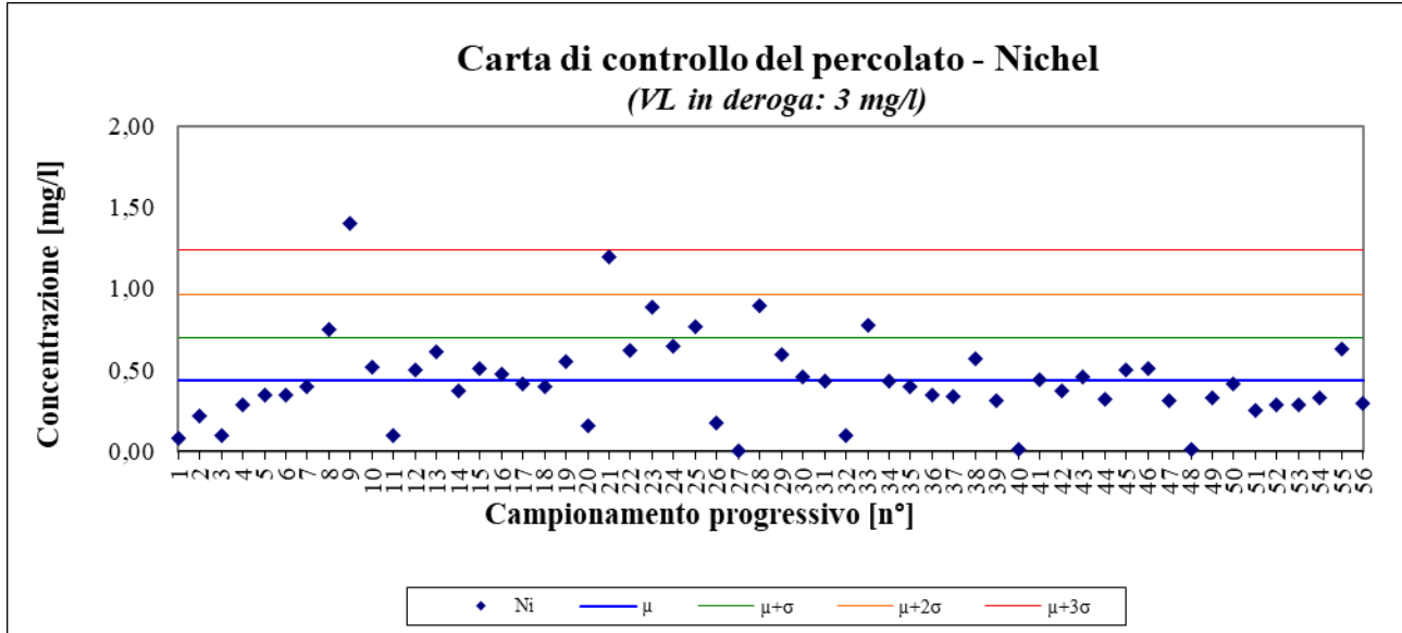
Figura 9 – Nichel; periodo gennaio 2010 – ottobre 2023
