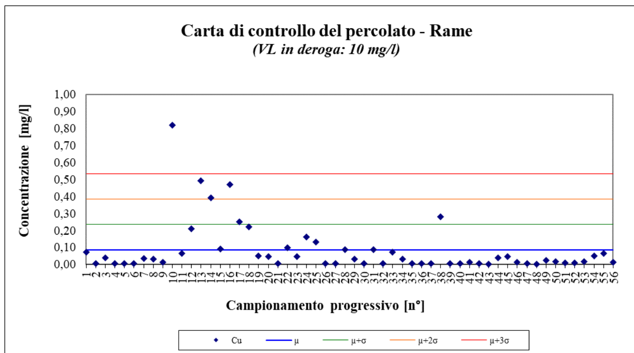
Figura 6 – Rame; periodo gennaio 2010 – ottobre 2023
