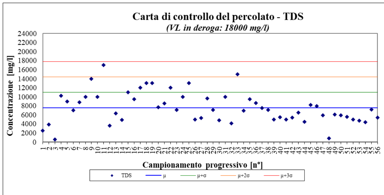
Figura 3 – TDS; periodo gennaio 2010 – ottobre 2023
