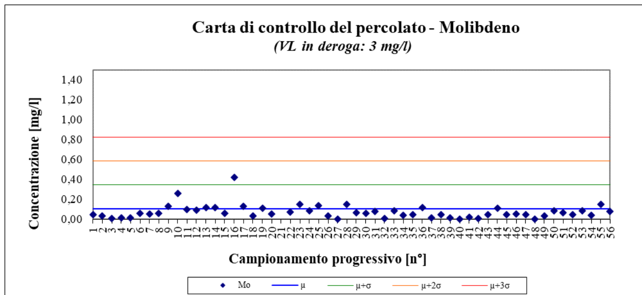
Figura 7 – Molibdeno; periodo gennaio 2010 – ottobre 2023
