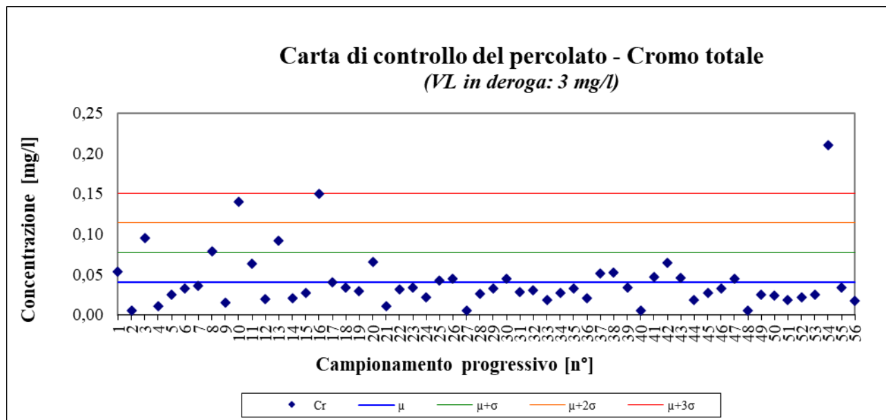
Figura 5 – Cromo totale; periodo gennaio 2010 – ottobre 2023
