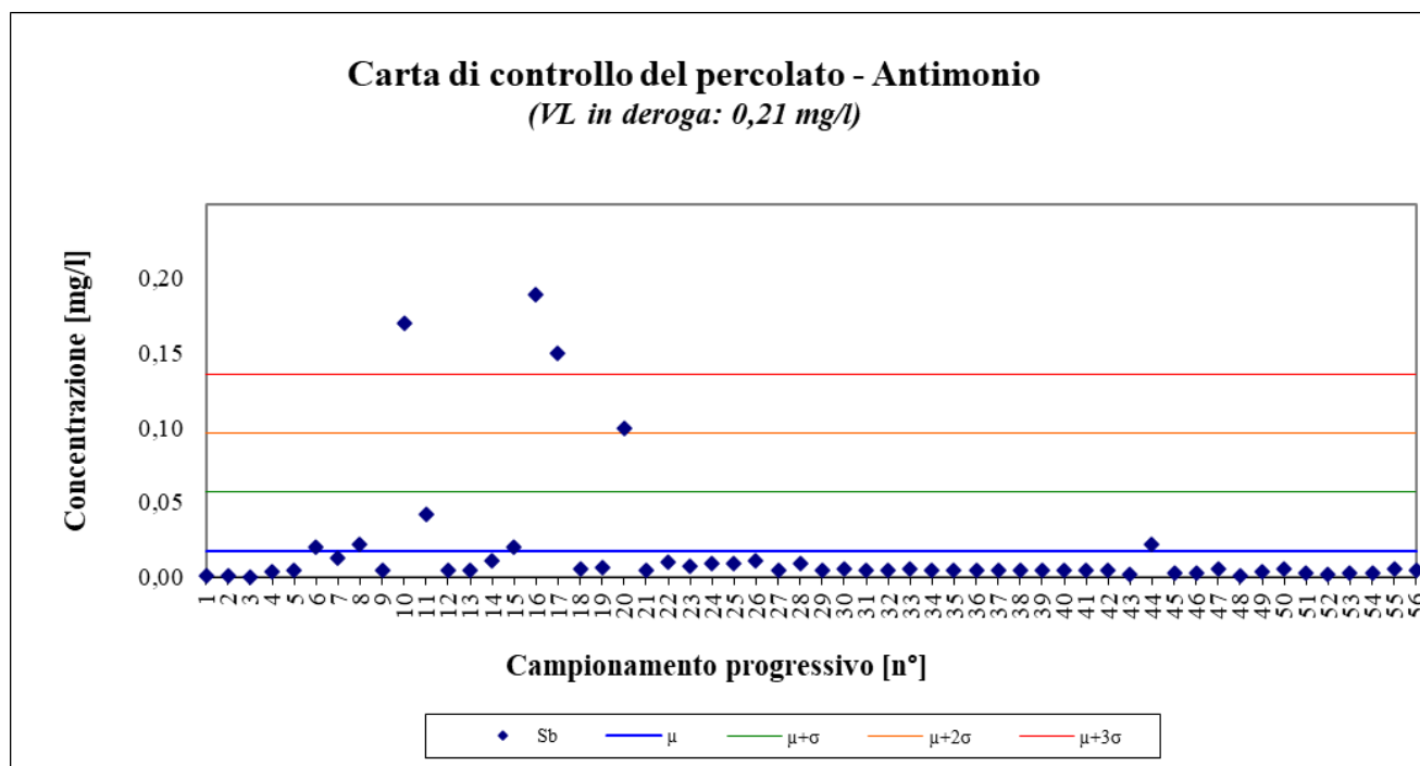
Figura 8 – Antimonio; periodo gennaio 2010 – ottobre 2023
