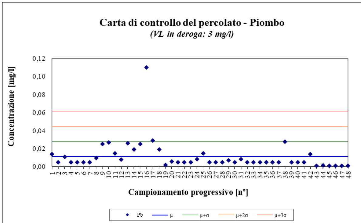
Figura 10 – Piombo; periodo gennaio 2010– ottobre 2021
