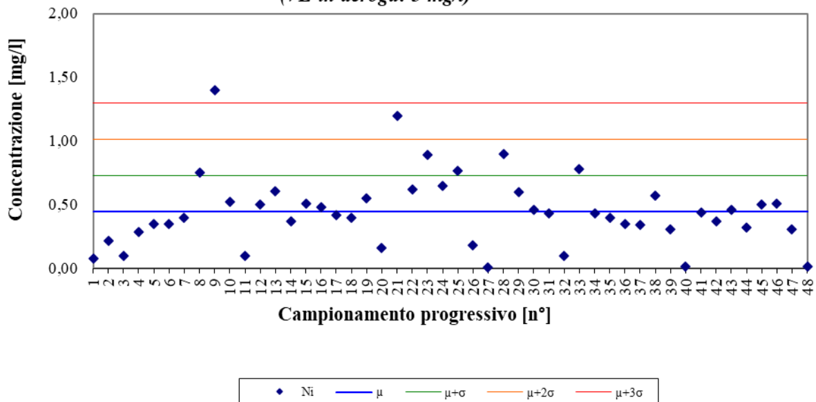
Figura 9 – Nichel; periodo gennaio 2010 – ottobre 2021
