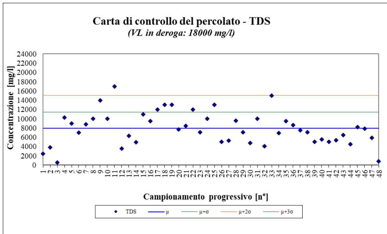
Figura 3 – TDS; periodo gennaio 2010 – ottobre 2021
