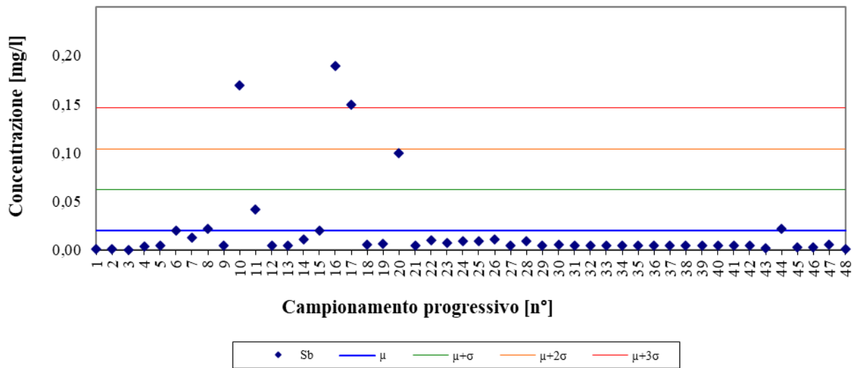
Figura 8 – Antimonio; periodo gennaio 2010 – ottobre 2021
