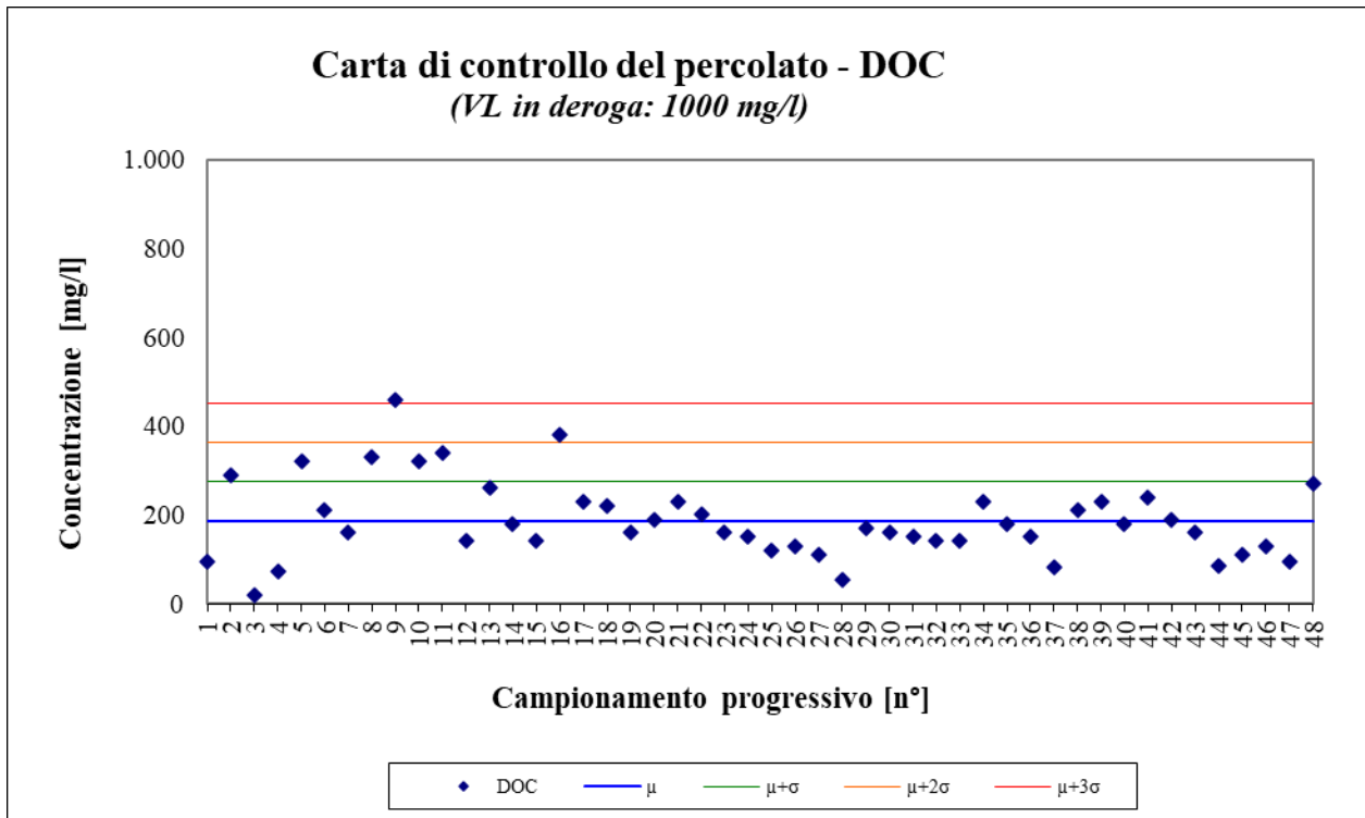
Figura 4 – DOC; periodo gennaio 2010 – ottobre 2021
