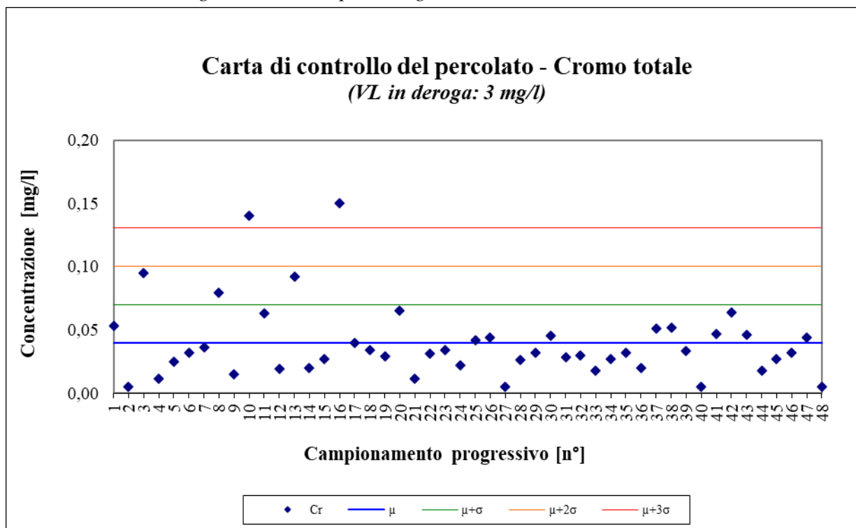
Figura 5 – Cromo totale; periodo gennaio 2010 – ottobre 2021
