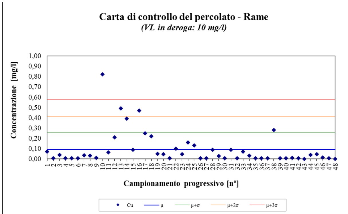
Figura 6 – Rame; periodo gennaio 2010 – ottobre 2021
