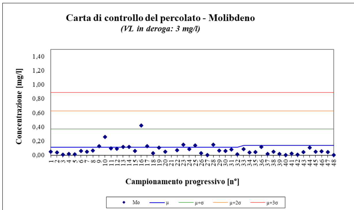
Figura 7 – Molibdeno; periodo gennaio 2010 – ottobre 2021
