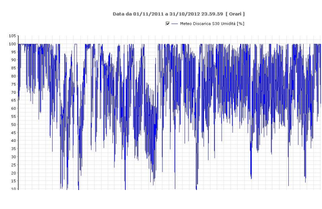
Figura 5: Andamento della umidità relativa [%]
