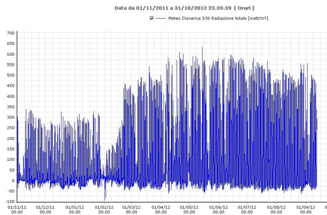
Fig. 6: Andamento della radiazione solare incidente [W/m²]
