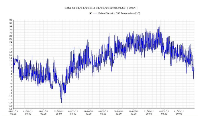
Figura 4: Andamento della temperatura [°C]
