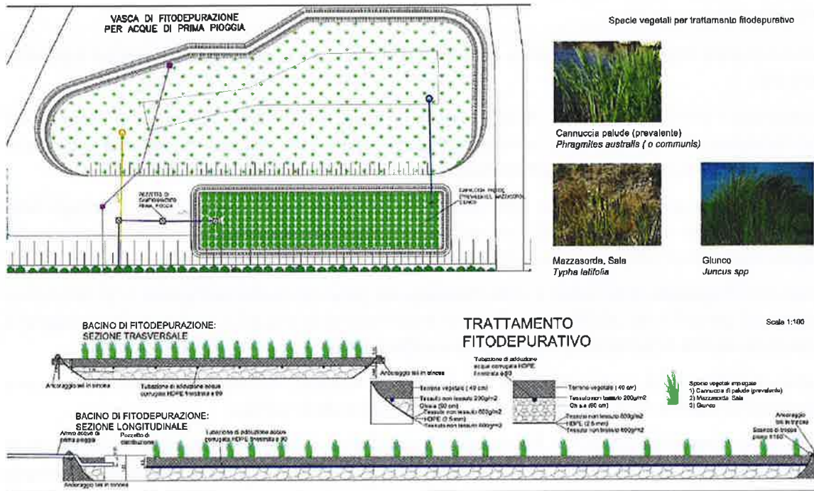
Fig. 5.6 – Fitoepotraspirazione per il trattamento delle acque di prima pioggia
