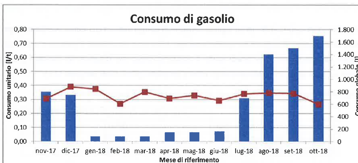
Fig. 12.7 – Istogramma consumi mensili di gasolio
