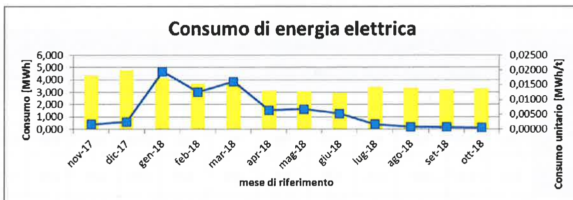
Fig. 12.5 – Istogramma consumi mensili di energia elettrica
