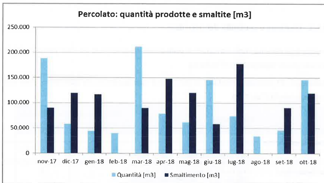
Fig. 13.9A – Quantitativi mensili di percolato prodotto e smaltito (novembre 2017-ottobre 2018)
