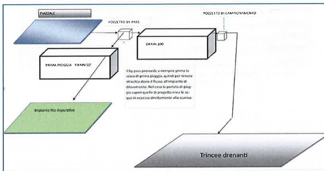
Fig. 13.5 - Schema a blocchi sistema di gestione acque meteoriche
