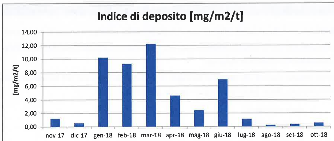
Fig. 12.13 - Andamento dell'indice di deposito
