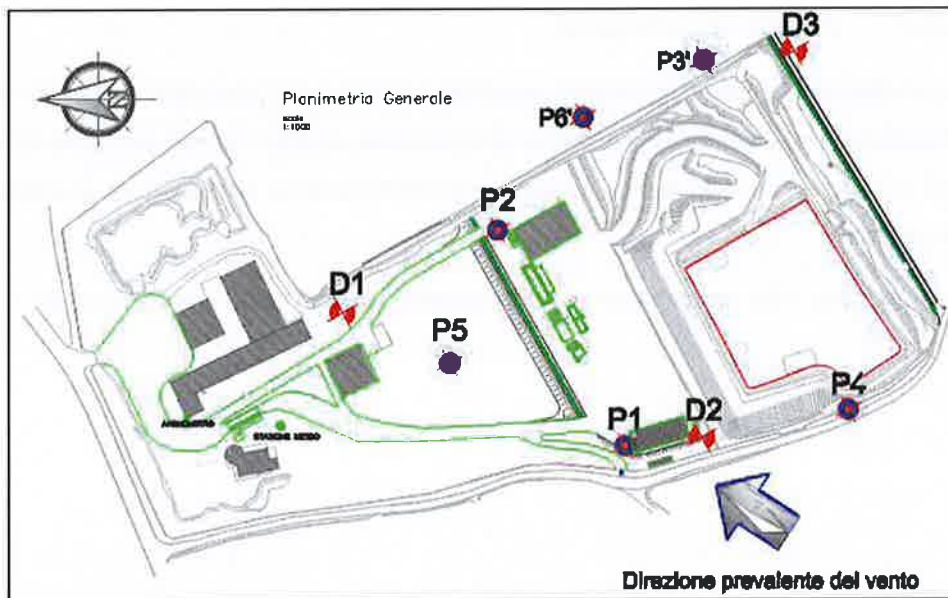
Fig. 13.12 – Planimetria con indicazione del posizionamento dei deposimetri: D1-D2-D3.
